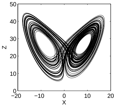
Fig. 2.5 Lorenz “butterfly” strange attractor. (J. Halcrow)
